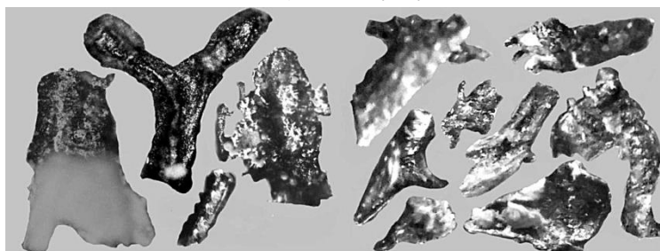
Рис.2. Осколки стримергласов кораллов, обнаруженные в Коралловой воронке (по [27]). (Поперечник снимка 2 мм)
