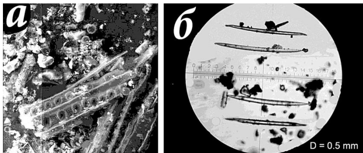
Рис.1. Стримергласы из грунтовых проб (по [20]): а – радиолярий (ширина снимка 150 мкм), б – спикул губок
