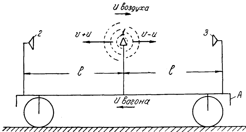
Рис. 8. Схема «опыта Майкельсона» для источника звука 1 и звукоприемников 2 и 3, движущихся относительно воздуха со скоростью u .
