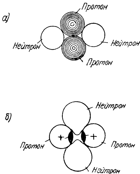
Рис. 2. Схемы строения ядра гелия.
