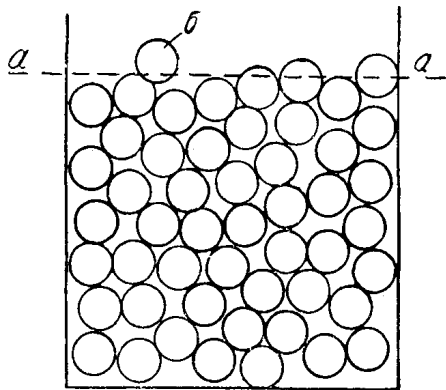
Рис. 4. Схематическое изображение микрообъема жидкости.
