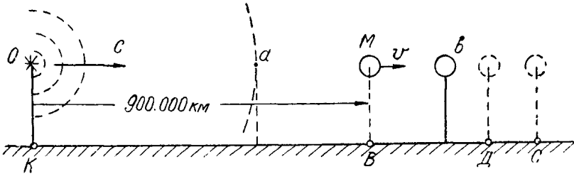
Рис. 9. Схема опыта, подтверждающая реальное существование относительной скорости c - v ( c — скорость распространения световой волны; v — скорость «убегания» тела M ).
