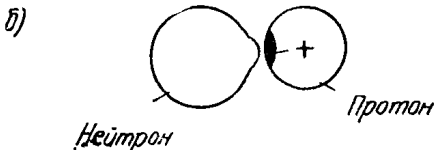
Рис. 1. Схемы строения ядра дейтрона.
