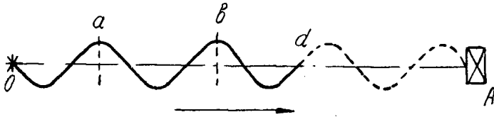
Рис. 6. Схематическое изображение монохроматической волны в момент начала ее распространения в среде с аномальной дисперсией (скорость распространения v > c ).
