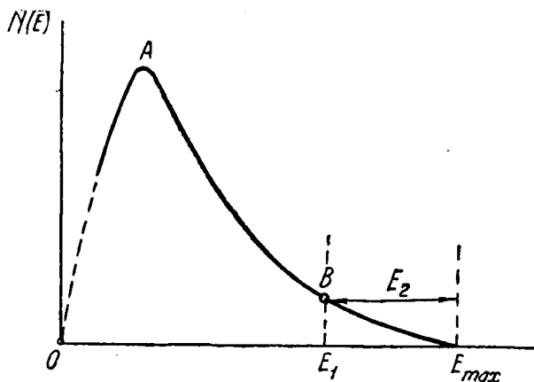
Рис. 3. Схема распределения энергии между бета-частицей и нейтрино согласно современной теории.
