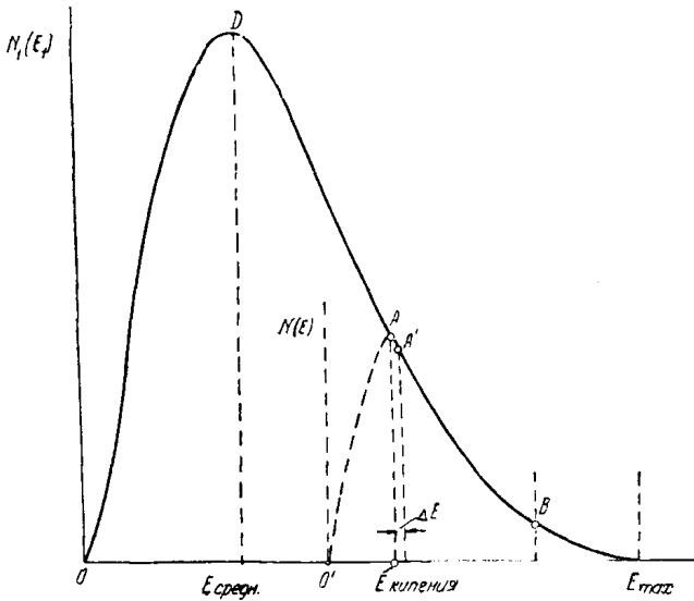
Рис. 5. Кривая распределения энергии частиц в жидкости ODE_{\text{max}} и кривая распределения энергии «испарившихся» частиц O'AE_{\text{max}} . Первая имеет начало координат в точке O , вторая — в точке O' .
